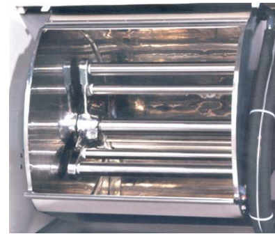
Type YY-3 agitator
